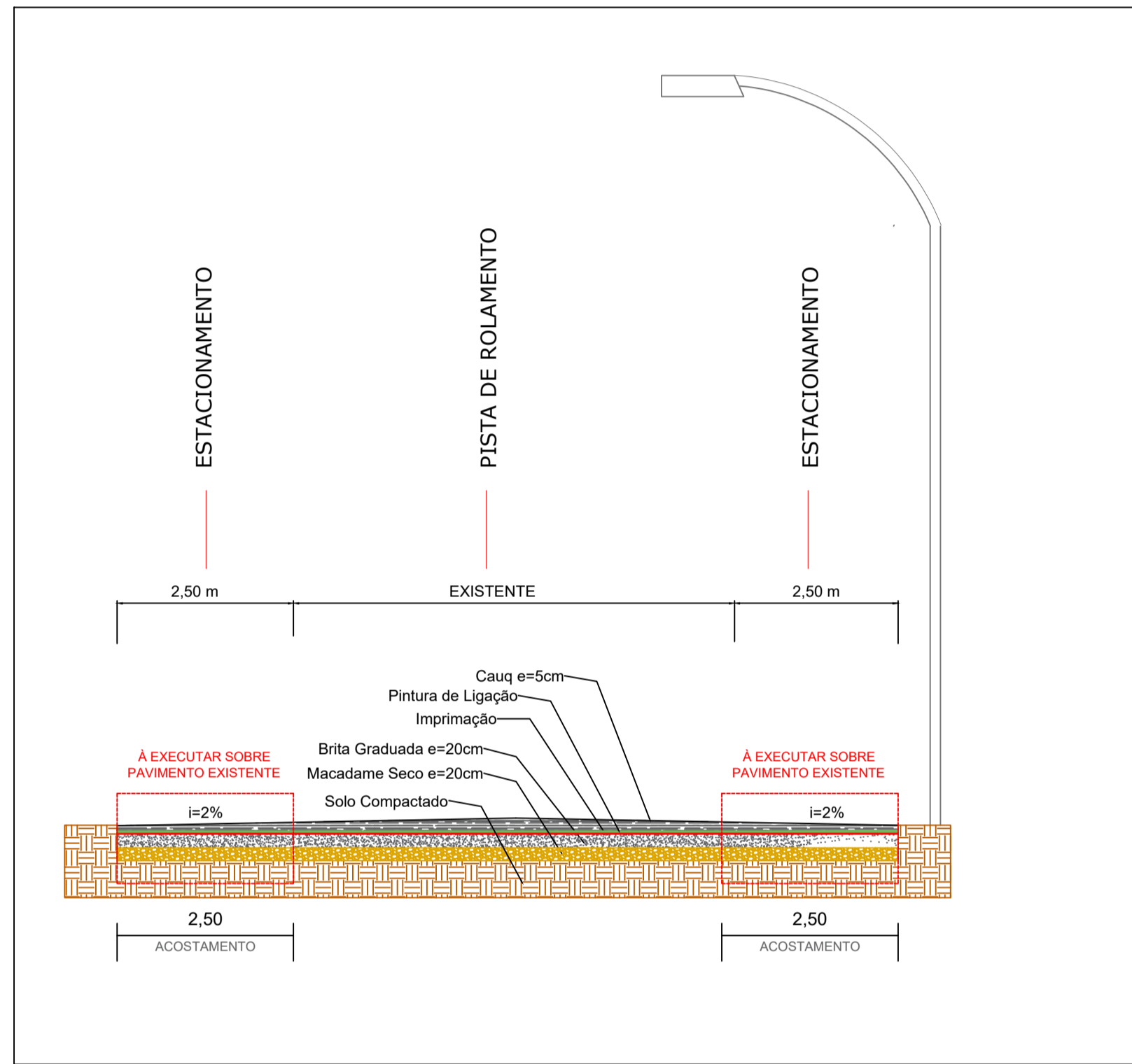
PERFIL TRANSVERSAL S/ESC
