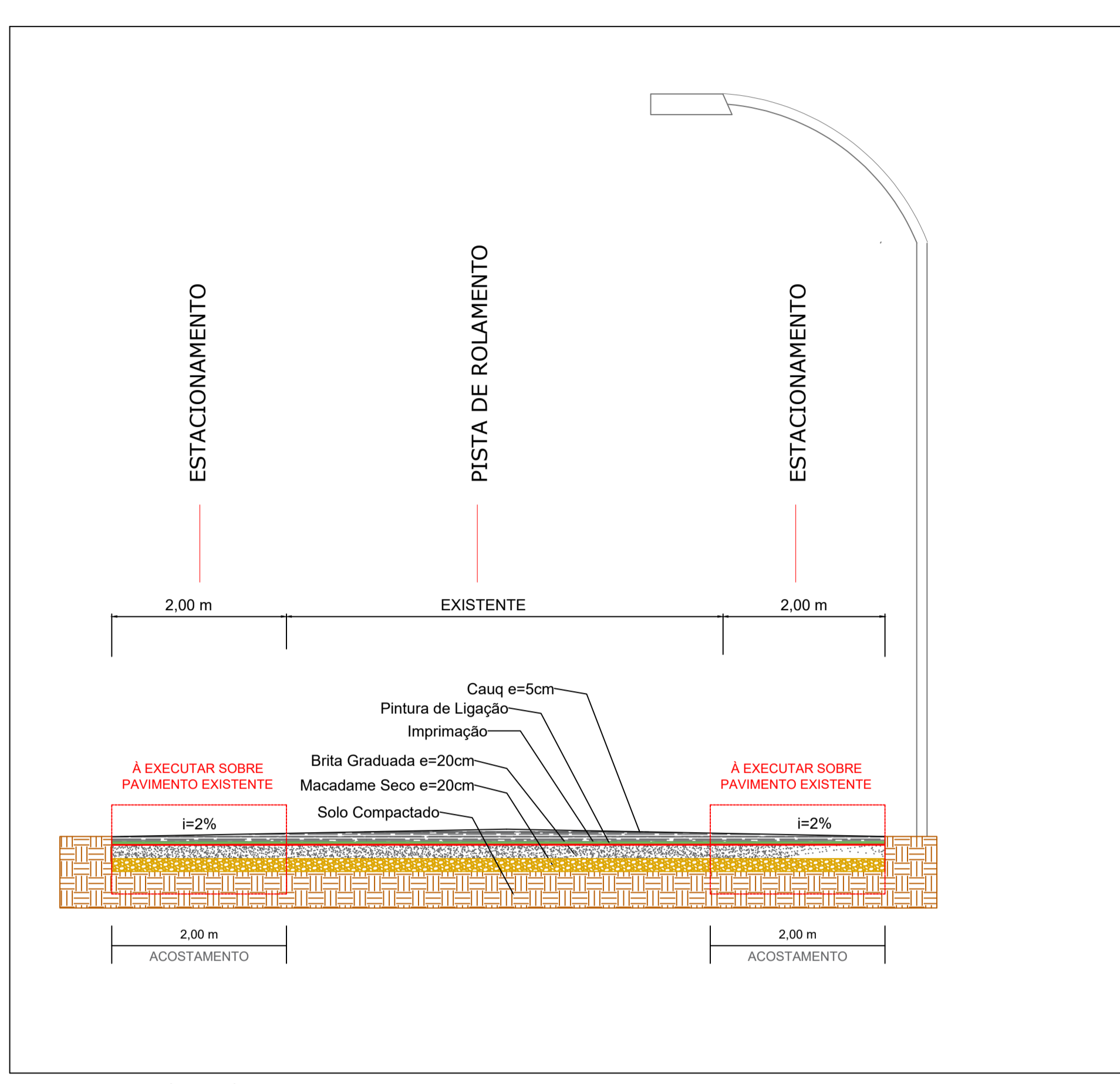
PERFIL TRANSVERSAL S/ESC
