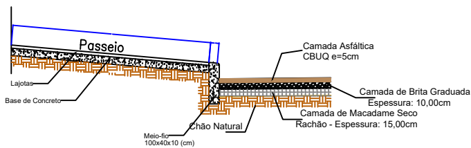
DETALHE MEIO-FIO Esc.: 1:20
