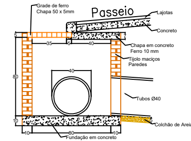
CAIXAS COLETORAS Sem Escala
