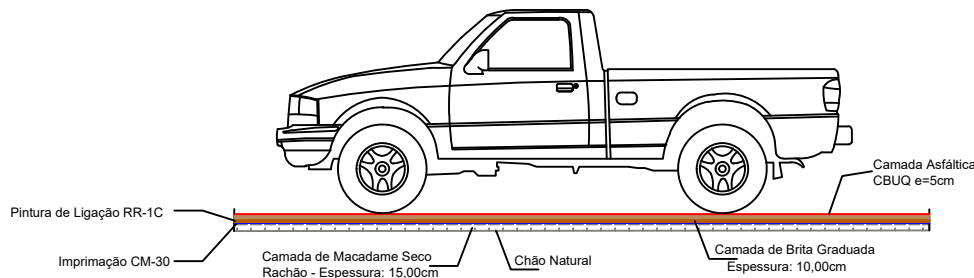
SEÇÃO TRANSVERSAL DA PAVIMENTAÇÃO ASFÁLTICA SOBRE CHÃO NATURAL
