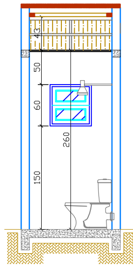
CORTE A-A'
