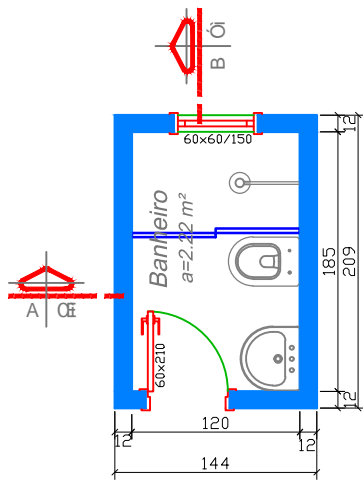
PLANTA BAIXA ÁREA= 3,01 m 2 ESCALA 1:50
