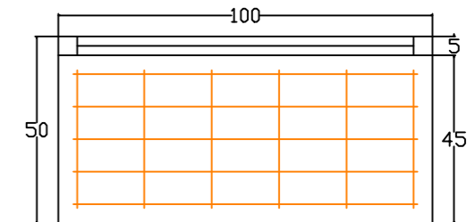
CHAPA DE CONCRETO FERRO 10 mm
