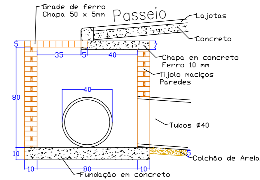
CAIXAS COLETORAS S/ Escala
