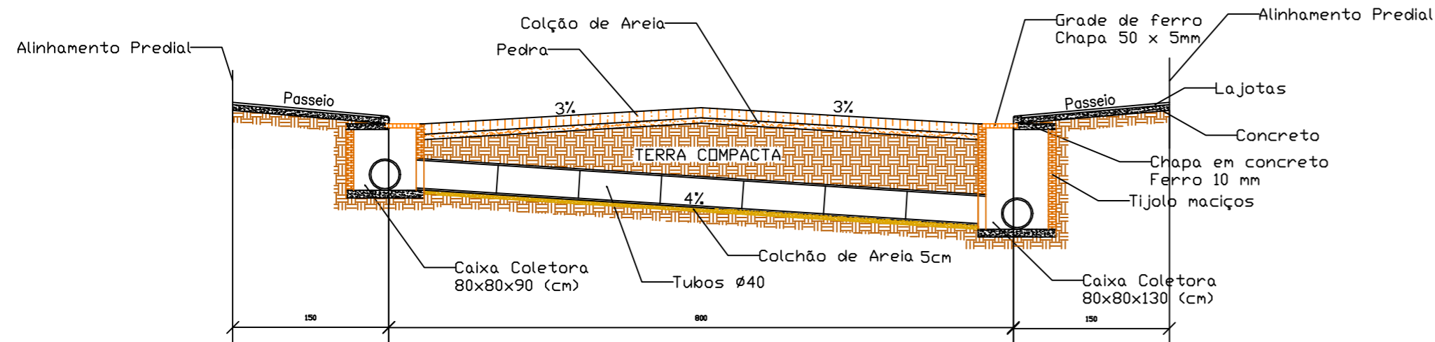
PERFIL TRANSVERSAL S/ Escala
