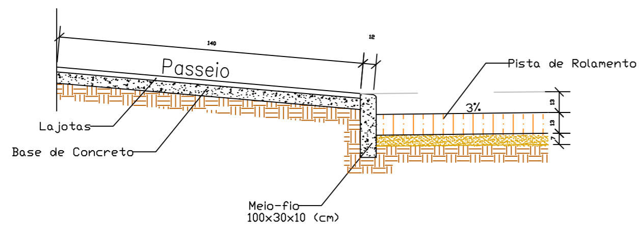
DETALHE MEIO-FIO Esc.: 1:20
