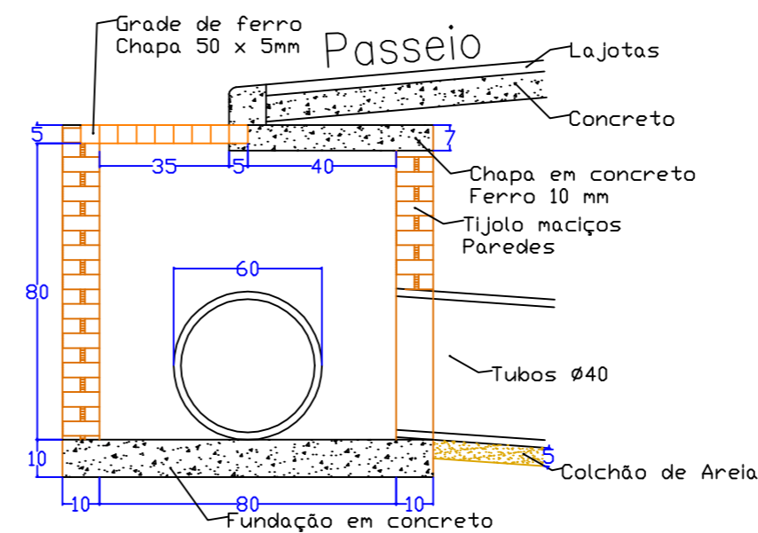
CAIXAS COLETORAS S/ Escala
