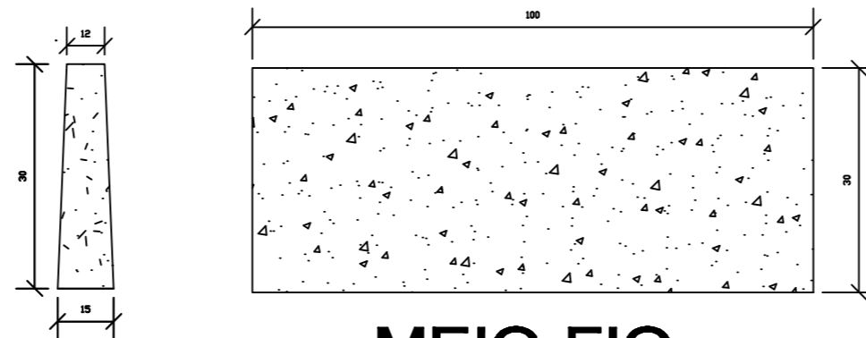
MEIO-FIO Esc.: 1:10
