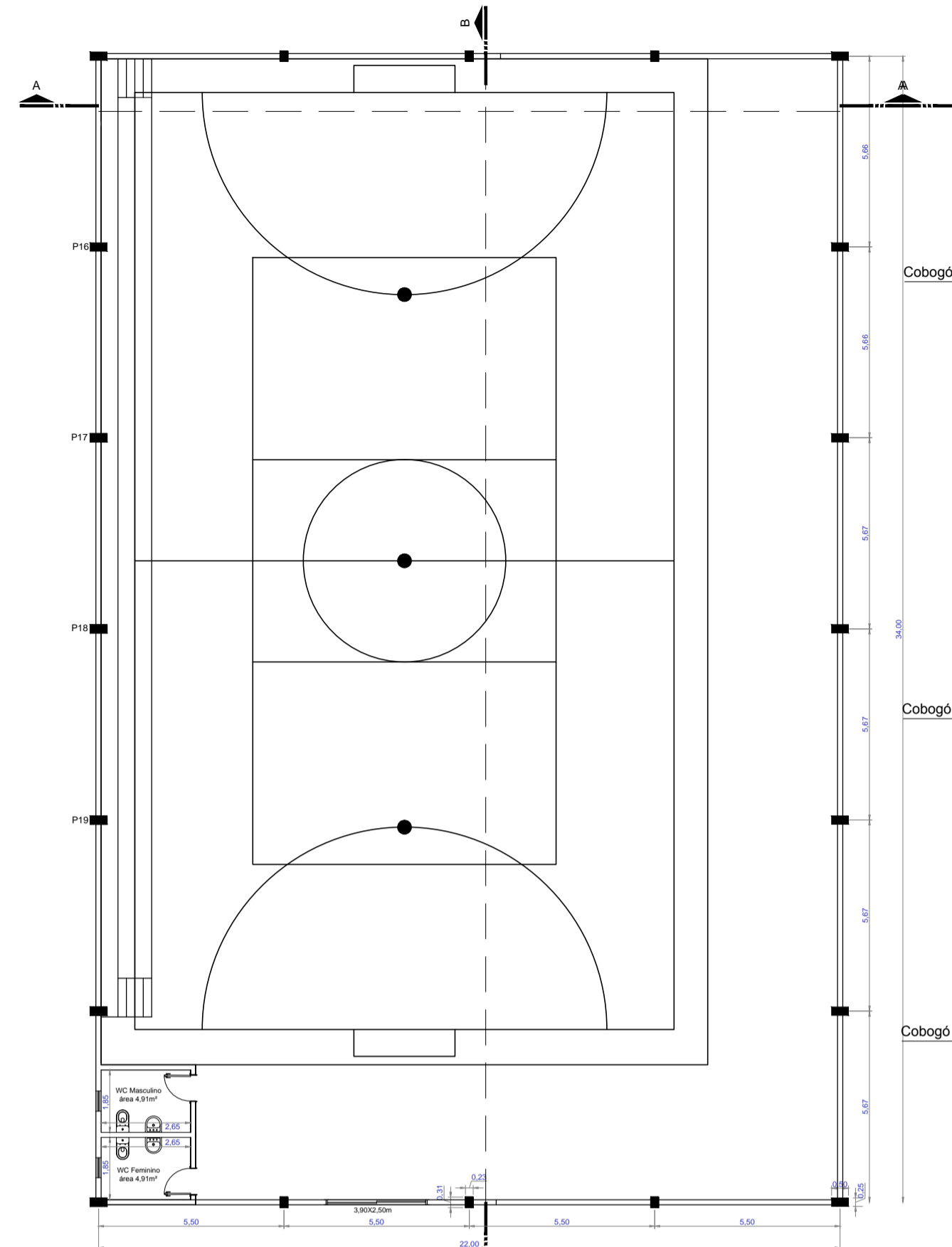
PLANTA BAIXA Área Construída: 756,42m² Escala: 1:150
