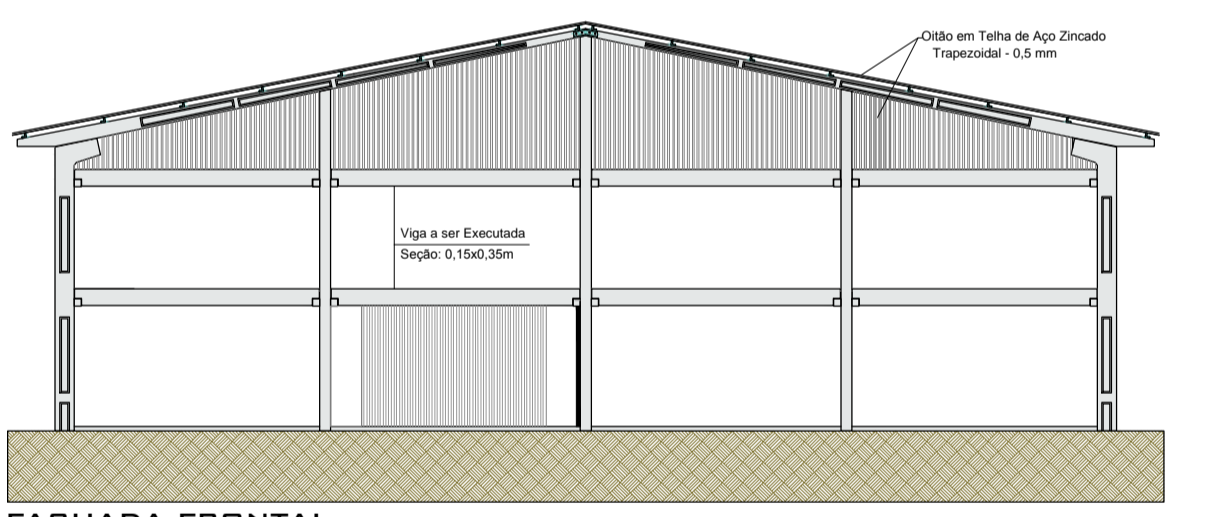
FACHADA FRONTAL Área Construída: 756,42m² Escala: 1:150
