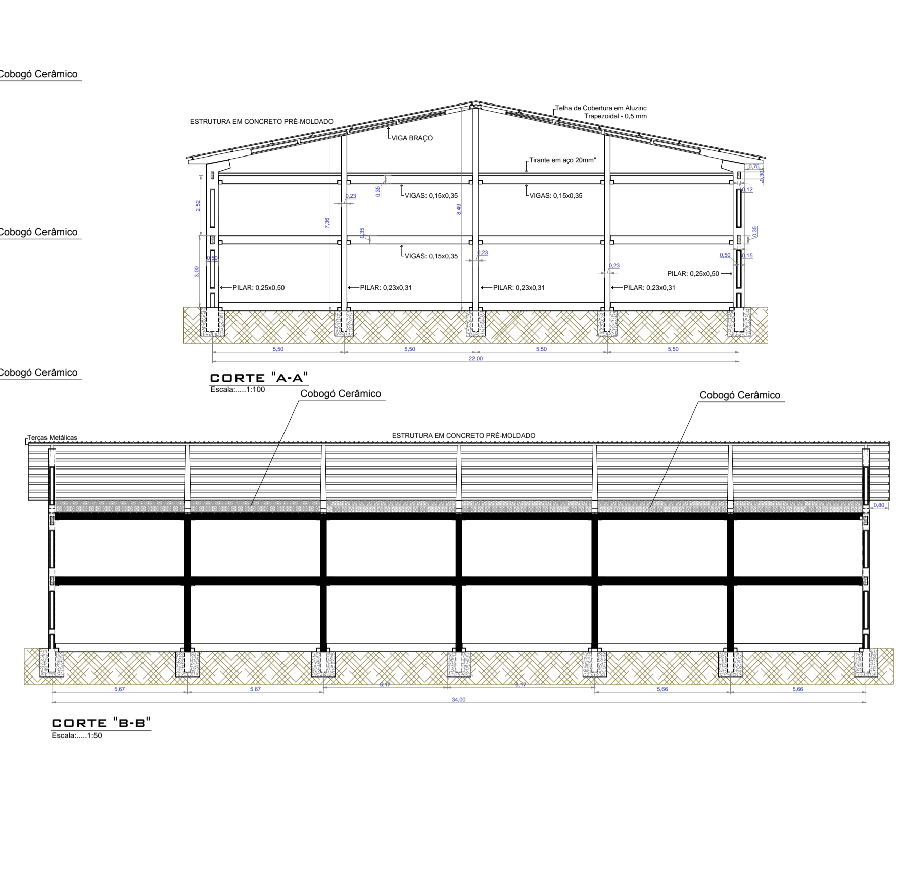
CORTE "A-A" Escala: 1:100
