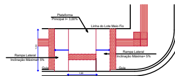
DETALHE DA RAMPA DE ACESSIBILIDADE CONFORME NBR - 9050/2015 Sem Escala
