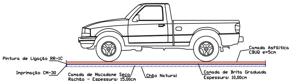
PERFIL TRANSVERSAL Sem Escala
