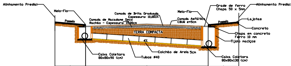
PERFIL TRANSVERSAL Sem Escala
