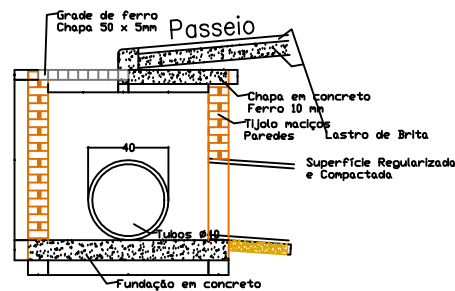
CAIXAS COLETORAS Sem Escala
