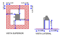
DETALHAMENTO DE OBSTÁCULOS Sem Escala
